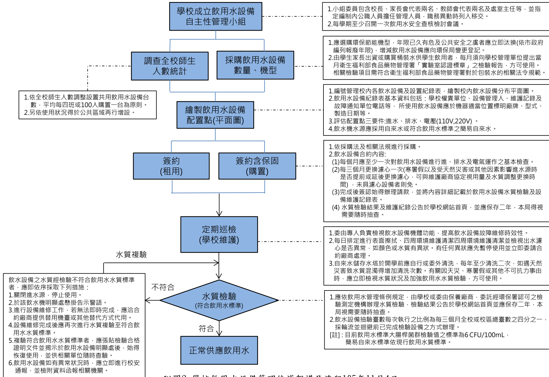
附圖2:學校飲用水設備管理維護架構及流程105年11月4日
